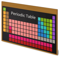
PeriodicTable
