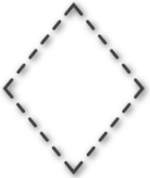
Area_Rhombus
